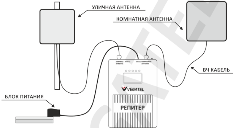
СХЕМА ПОДКЛЮЧЕНИЯ РЕПИТЕРА
